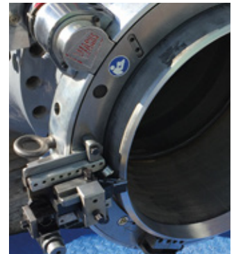
Pipe Beveling
